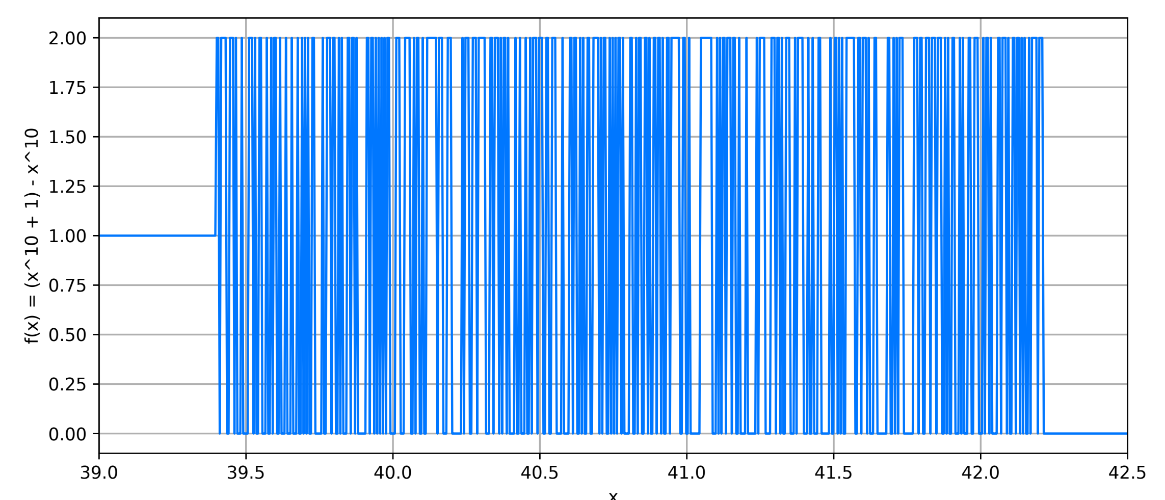
Figura 2: Resultado da avaliação da função f(x) = x^{10} + 1 - x^{10} num SPF IEEE de 64 bits. Fonte: Autor.
