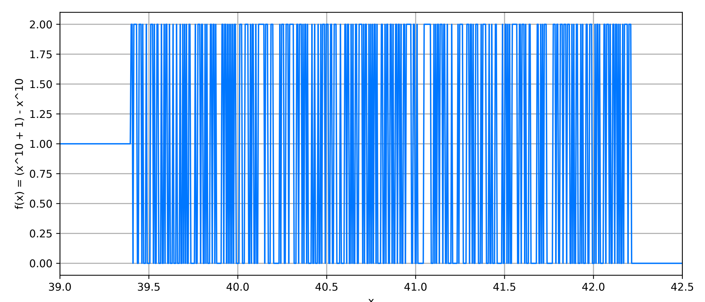
Figura 3: Resultado da avaliação da função f(x) = x^{10} + 1 - x^{10} num SPF IEEE de 64 bits. Fonte: Autor.
